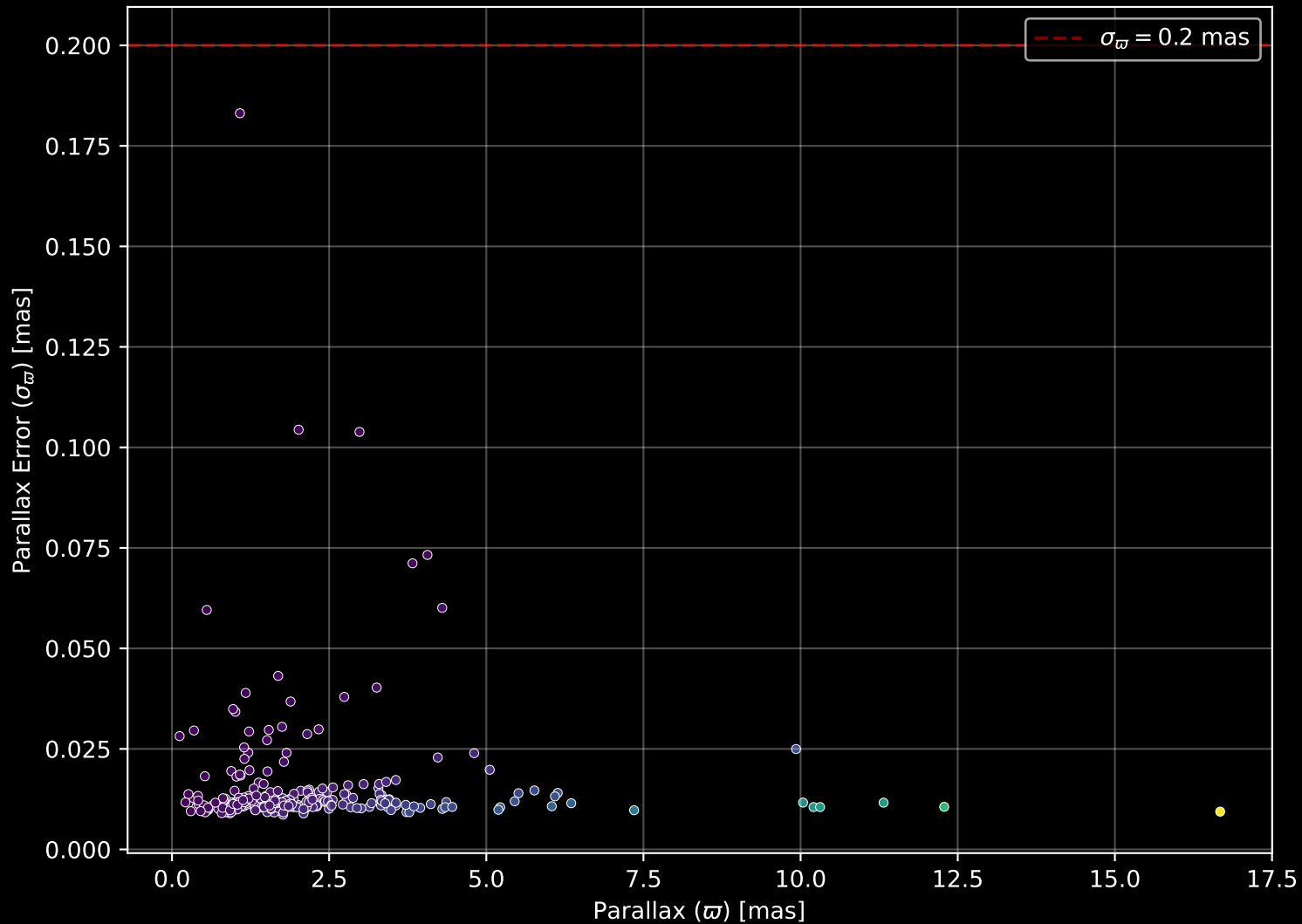
GALAH DR4 Field: [7144] Parallax Quality (n= 255)
