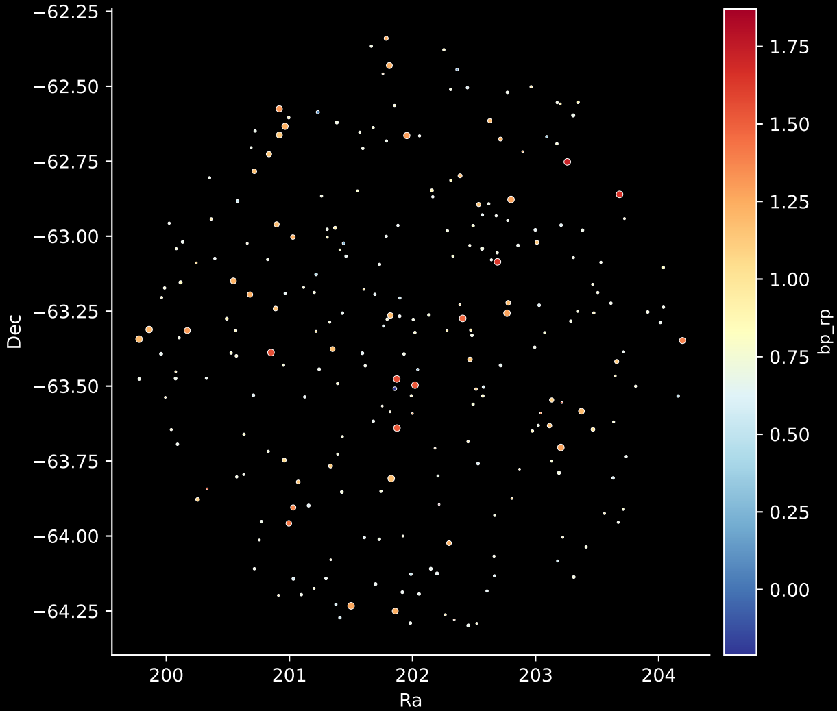
GALAH DR4 Field: [7144] Stars: 255
