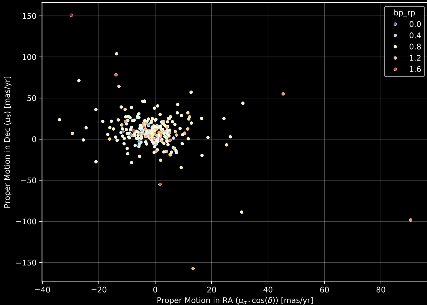
GALAH DR4 Field: [7144] Proper Motion Diagram (n= 255)
