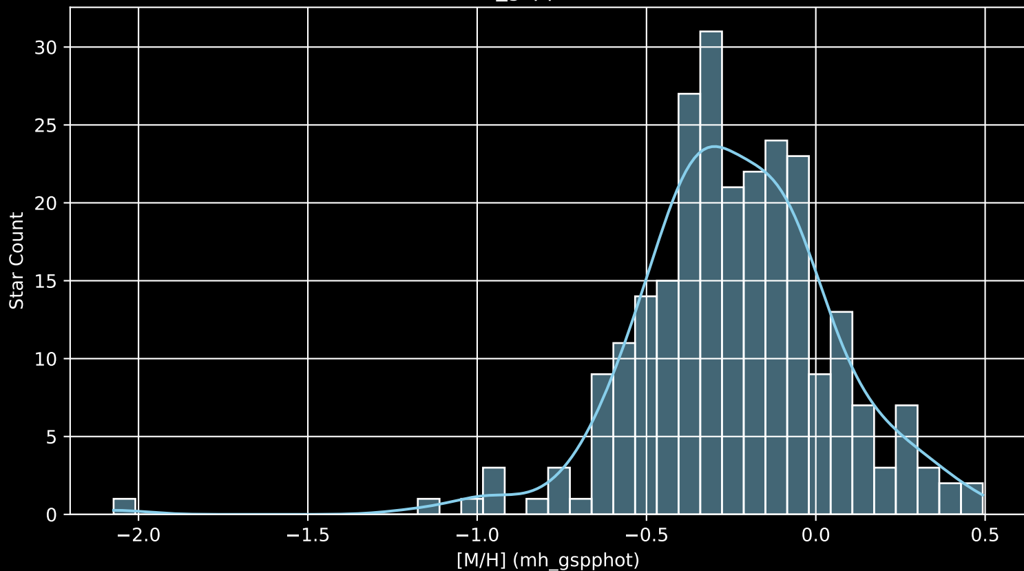
GALAH DR4 Field: [7144] [M/H] (mh_gspphot) (n= 254)
