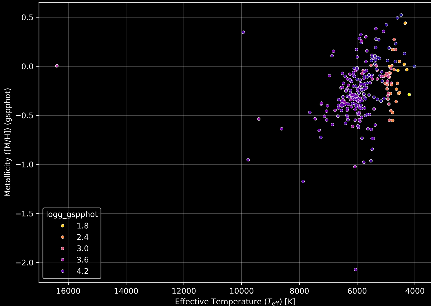
GALAH DR4 Field: [7144] Stellar Population Parameters (n= 255)
